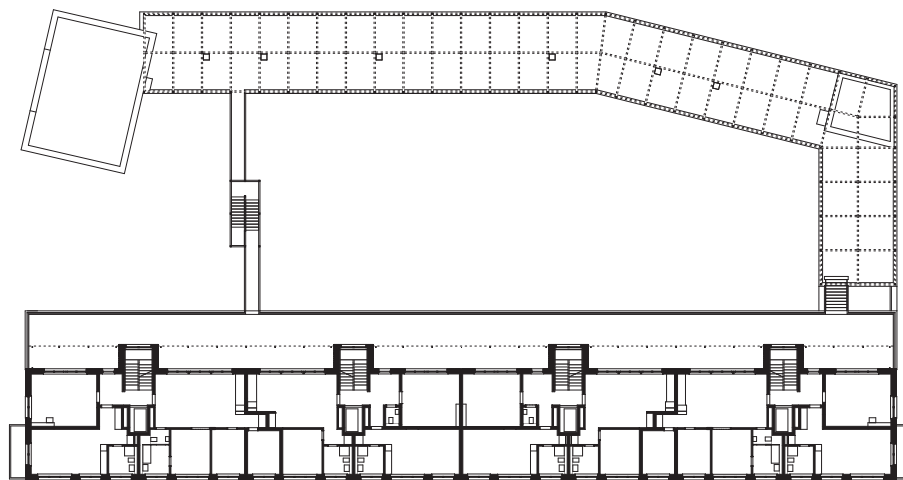
4. Obergeschoss mit Dachterrasse
