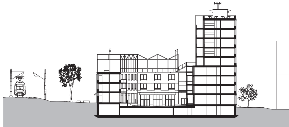
Querschnitt
