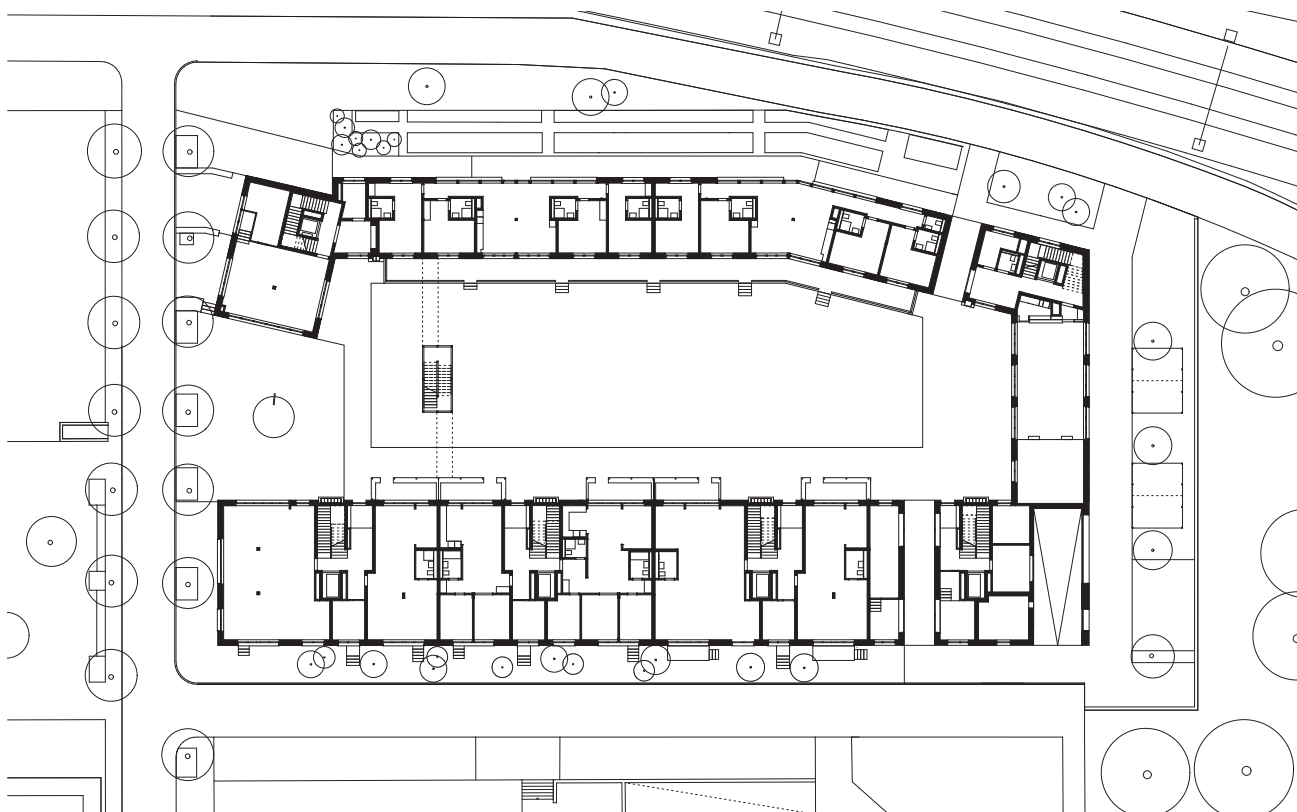
Erdgeschoss mit Umgebung
